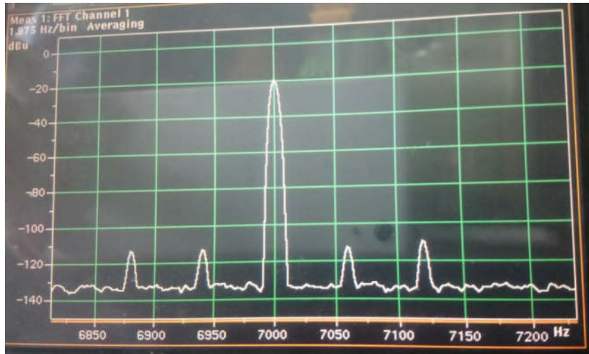
График интермодуляционных искажений плеера тест SMPTE
