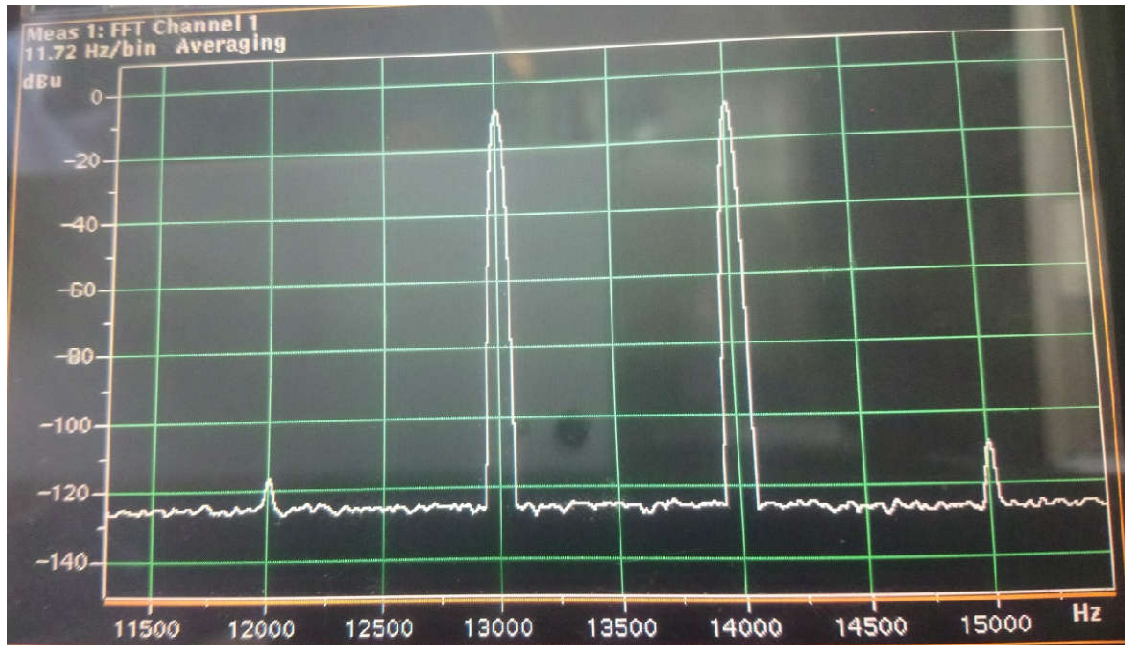
График интермодуляционных искажений.
