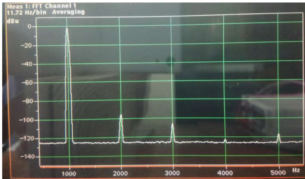
Спектр выходного сигнала плеера частотой 1 кГц.
