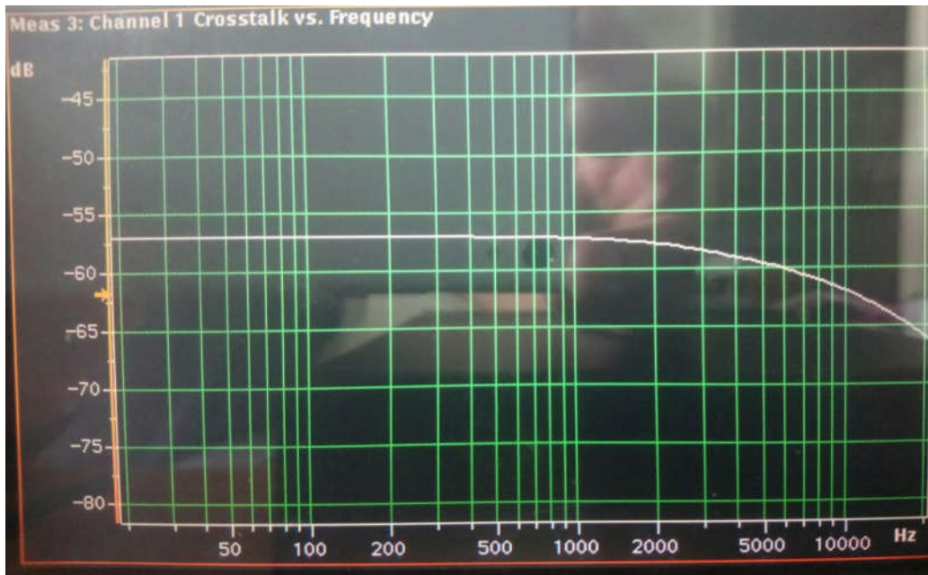
График характеристики разделения стерео каналов Разделение стереоканалов составляет -56 дБ на частоте 1000 Гц.
