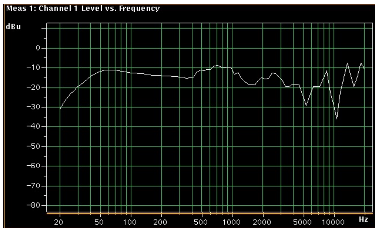
АЧХ наушников в звуковом диапазоне
