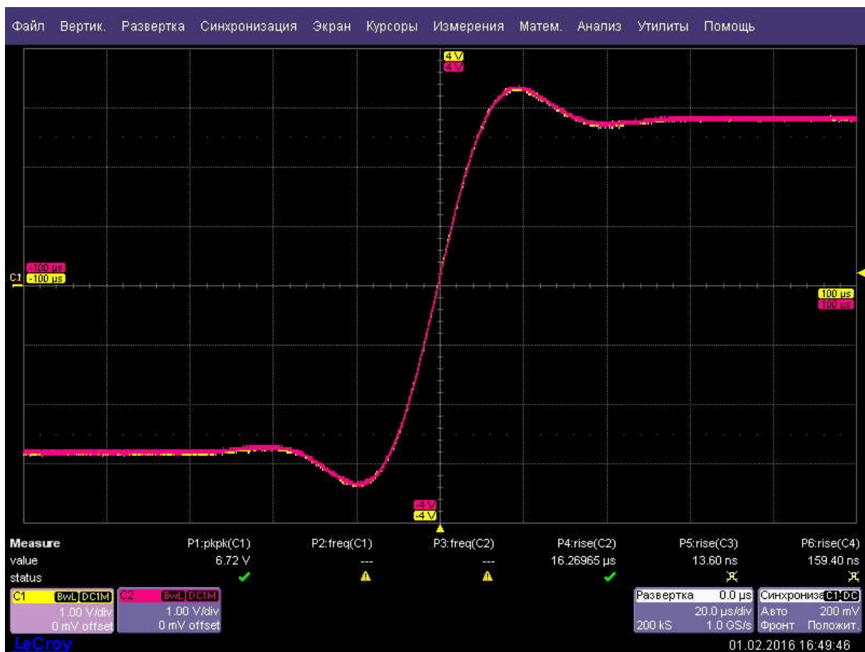
График фронта прямоугольного сигнала. Длительность фронта составляет 20 микросекунд.
