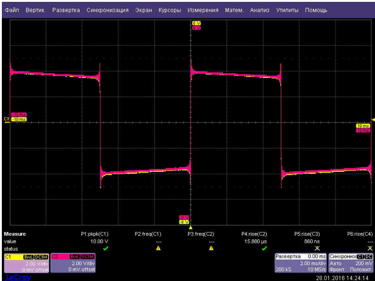
График выходного сигнала прямоугольной формы частотой 100 Гц. Присутствуют выбросы.
