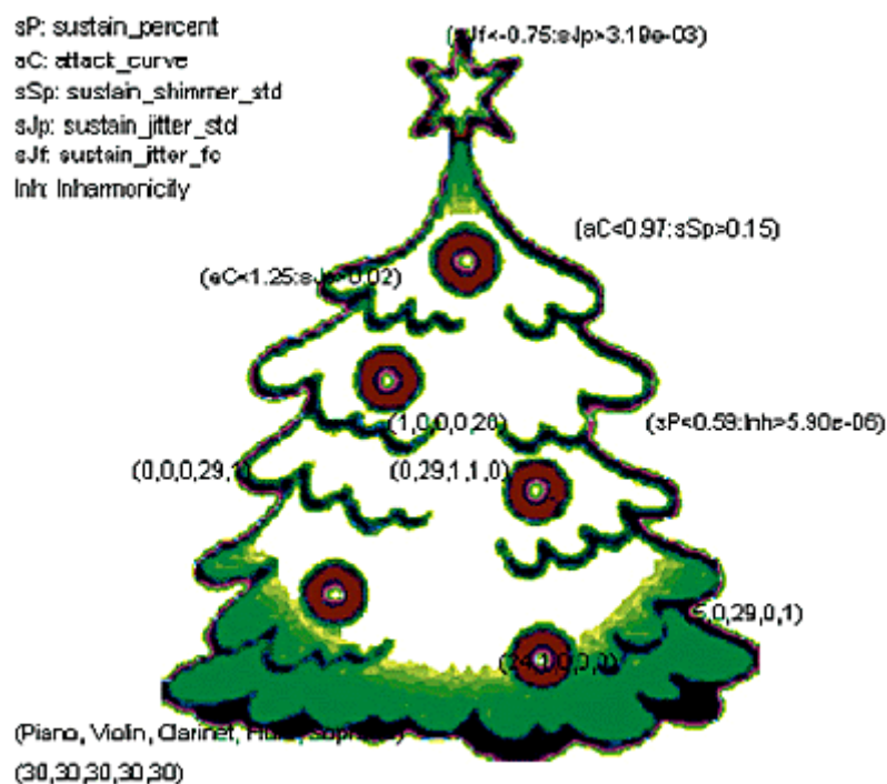
Рис. 5 "Бинарное дерево"
