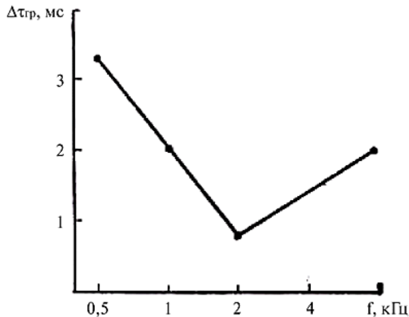
Рис. 1 Зависимость порогов слышимости искажений ГВЗ от частоты
